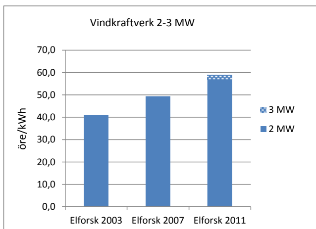
Figur 2.4.3 Produktionskostnader för medelstora vindkraftverk (2-3 MW) på land enligt Elforks rapportserie El från nya anläggningar åren 2003, 2007 och 2011, 2010 års priser. Källa: Elforsk
