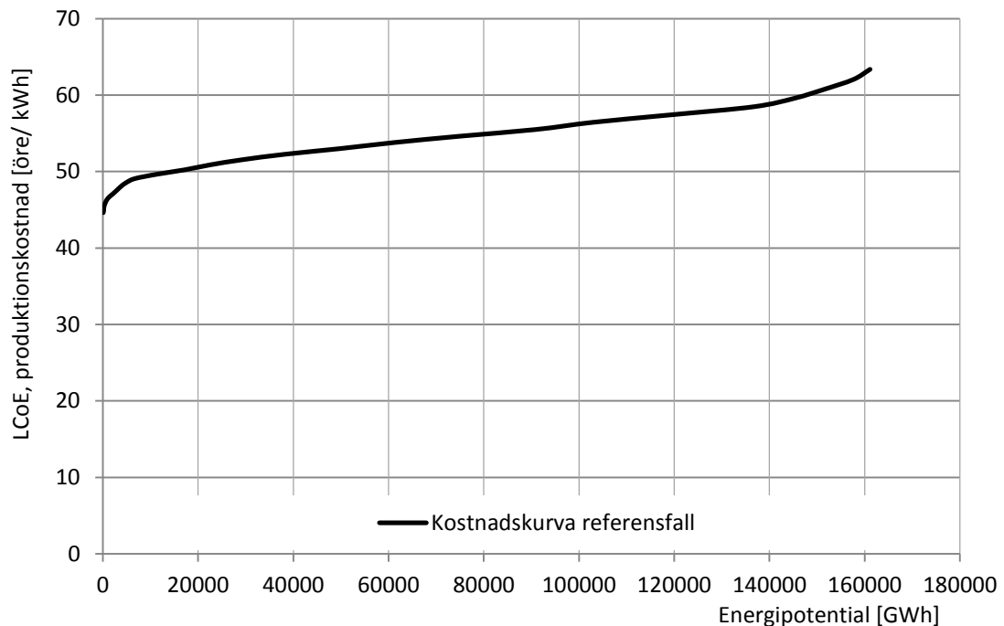
Figur 4.1.1 Kostnadskurva för svenska vindkraftsprojekt.
