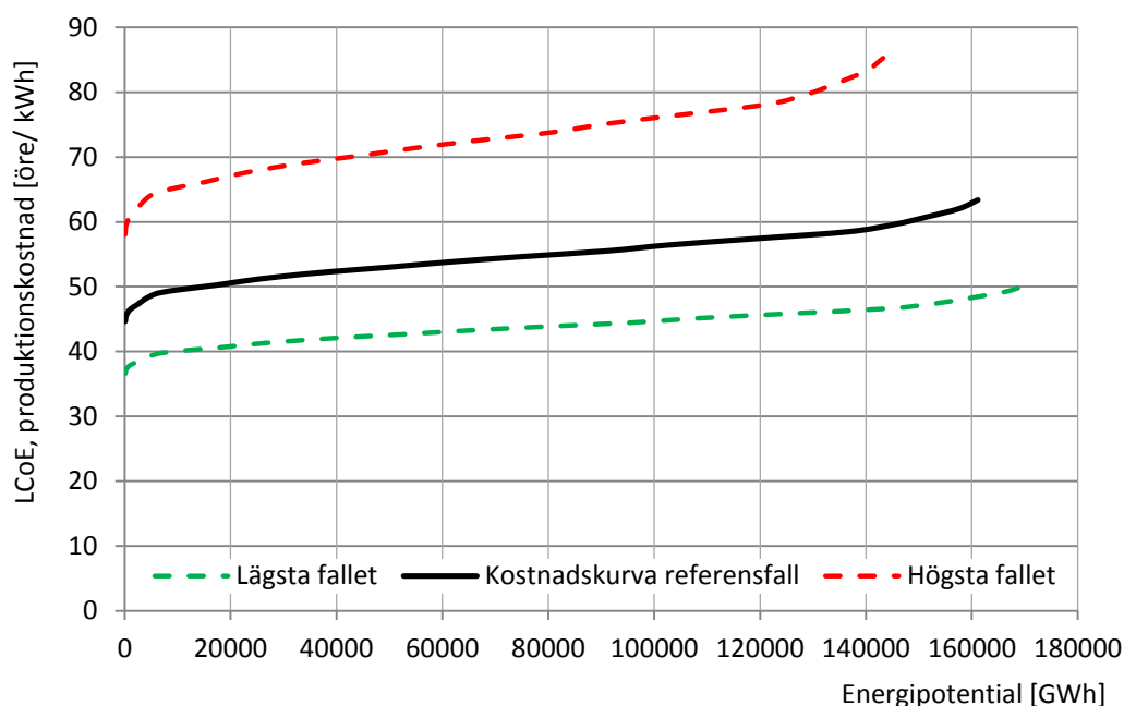
Figur 5.1.1 Kostnadskurva för vindkraftprojekt i Sverige inklusive lägsta och högsta fallet, d.v.s. utfall vid antagande om de mest respektive minst gynnsamma förhållandena.
