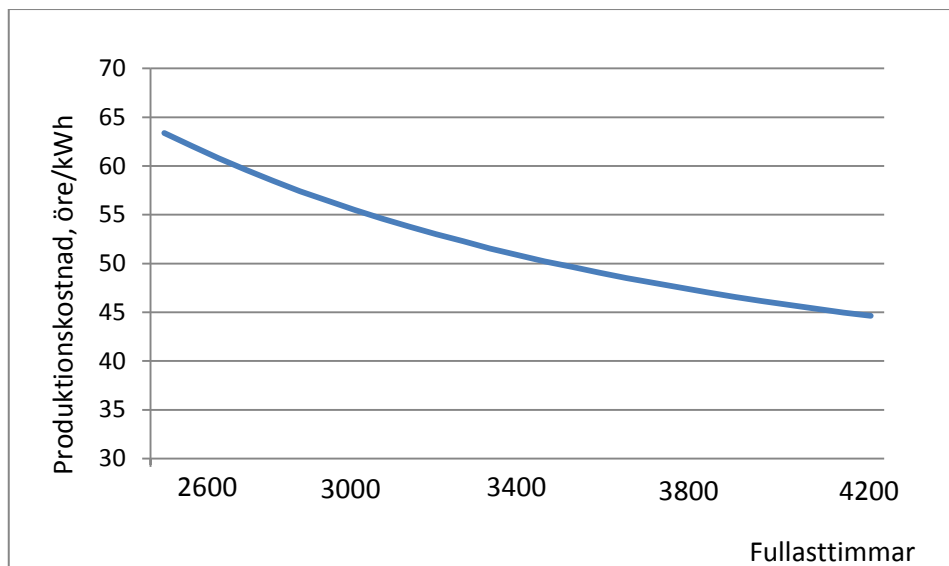
Figur 2.2.2 Beräknad produktionskostnader för vindkraft i Sverige, som en funktion av antalet fullasttimmar. Anm: I beräkningarna utgår från antagande om en klass II turbin 3,2 MW, de totala investeringskostnaderna sätts till 12000 kr/kW, drift och underhållskostnaderna 15 öre/kWh och kalkylräntan är 8 % och livslängden 20 år.
