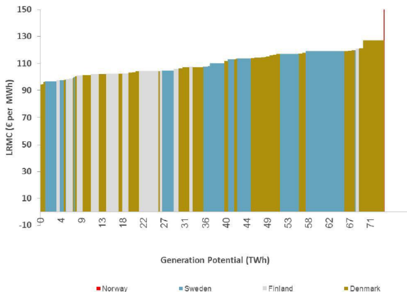
Figur 2.4.7. Långsiktig marginalkostnad, LRMC eller LCoE för nordiska projekt för havsbaserad vindkraft. Källa: Thema Consulting Group.
