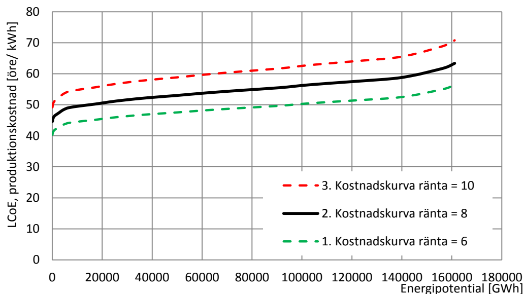
Figur 4.2.1 Produktionskostnaden för olika antaganden om kalkylränta. Detta styr tillsammans med den ekonomiska livslängden de skattade kapitalkostnaderna.
