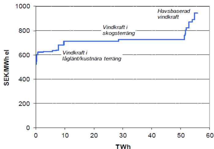
Figur 2.4.6 Utbudskurva för ny vindkraft i Sverige för modellår 2016 och framåt. Källa: Beräkningar med Markal-Nordic inför Långsiktsprognos 2012, Profu 2013.
