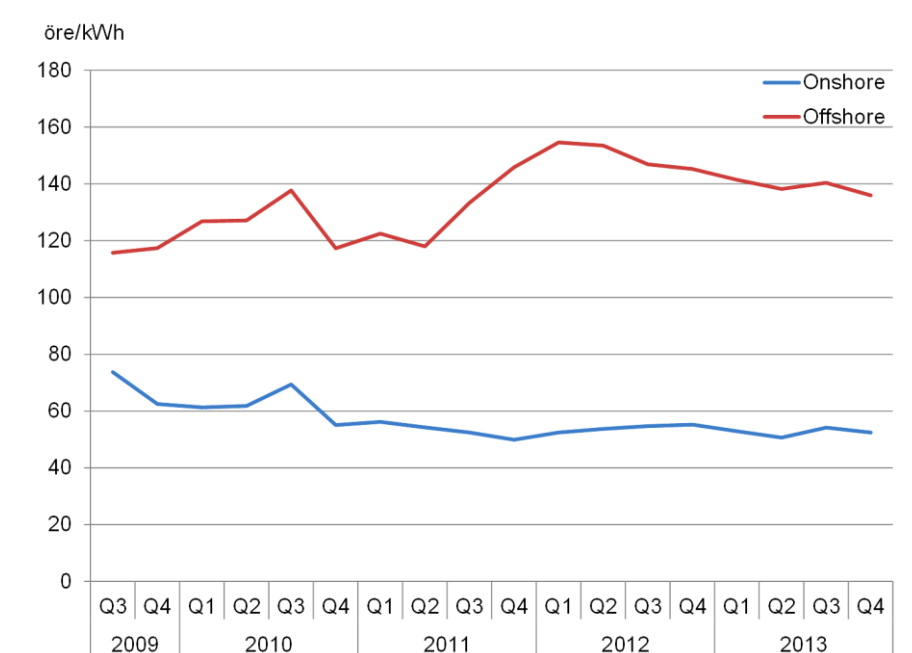
Figur 2.3.3 Utveckling av produktionskostnader för vindkraft i världen 2009-2013, öre/kWh, löpande priser. Källa: BNEF 2014
