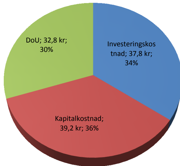
Figur 4.1.2 Fördelning av de totala kostnaderna för vindkraftprojektet i referensfallet. Investering på 12 Mkr/ MW på en 3,15 MW-turbin, kalkylränta 8 % och ekonomisk livslängd 20 år. Drift och underhållskostnad skattas till 15 öre/ kWh för en produktion motsvarande 3400 fullasttimmar om året under 20 år.
