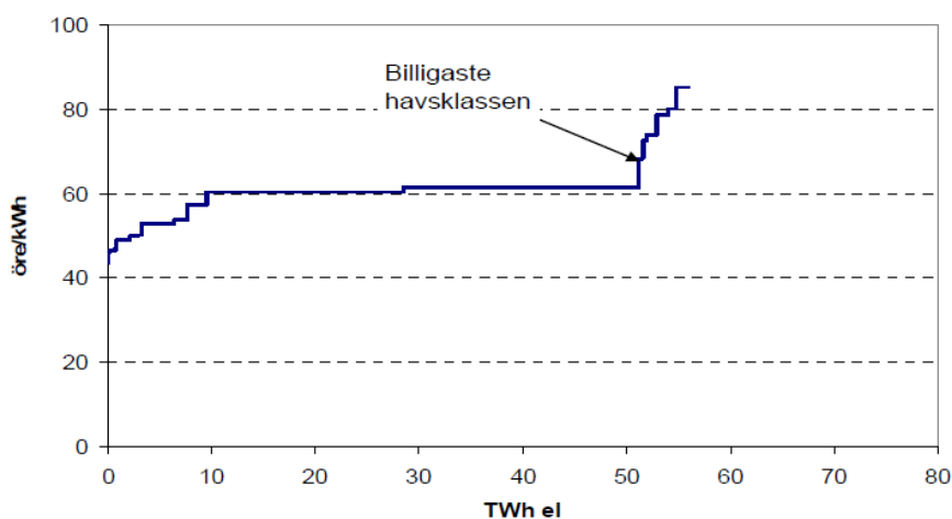
Figur 2.5.1 Produktionskostnad och potential för vindkraft. Figur från ”Samarbetsmekanismer enligt EU:s förnybartdirektiv”, ER 2010:18. Kostnaderna är inte uppdaterade för dagens turbiner. Källa: Vindkraft i framtiden, Elforsk 2008.
