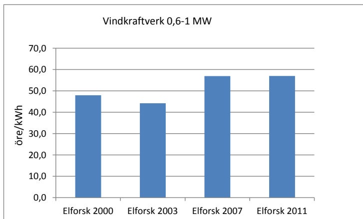
Figur 2.4.2 Produktionskostnader för mindre vindkraftverk (0,6-1 MW) på land enligt Elforks rapportserie El från nya anläggningar åren 2000, 2003, 2007 och 2011, 2010 års priser. Källa: Elforsk
