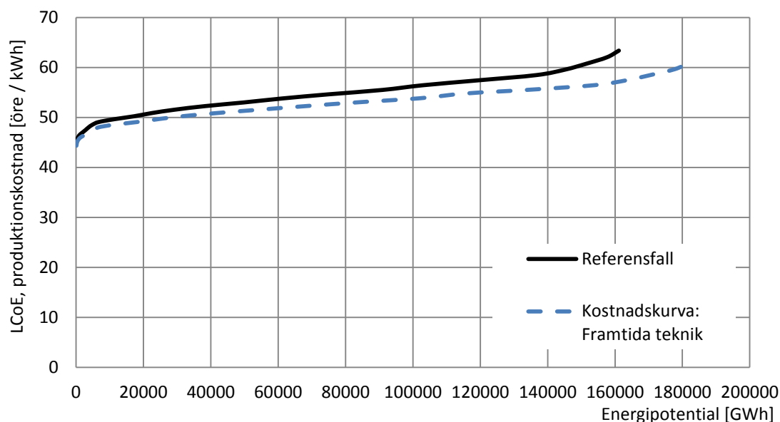
Figur 4.2.6 Kostnadskurva för referensfallet jämte kostnadskurvan för de antaganden som gjorts om teknikutveckling. Trots högre specifik investeringskostnad p.g.a. sjunkande effekt densitet (större turbin på given generator) ligger den framtida kostnadskurvan både lägre och sträcker sig längre än referensfallets. I övrigt är antaganden samma.
