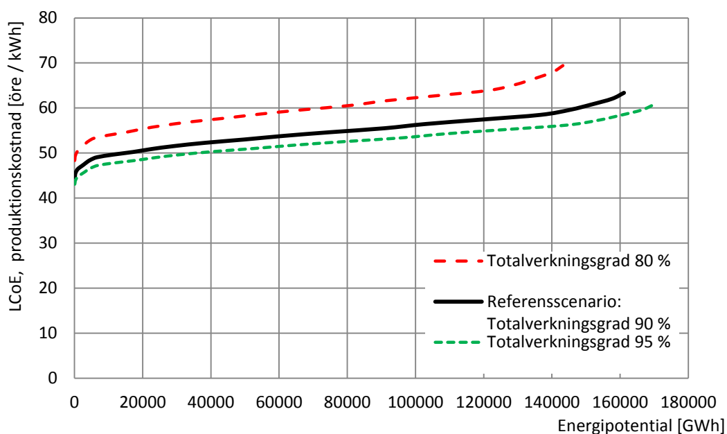
Figur 4.2.5 Produktionskostnaden för olika antaganden om projektportföljens verkningsgrad. Antagandet om projektens verkningsgrad påverkar driftekonomin men även den tillgängliga potentialen.
