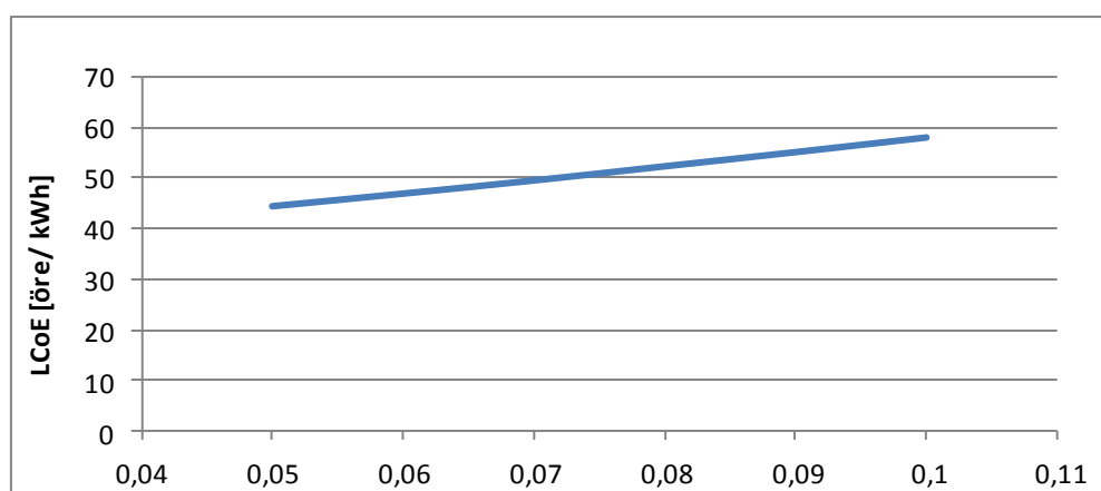
Figur 4.2.2 Grafen visar hur produktionskostnaden LCoE [kr/kWh] varierar för olika räntor (allt annat lika). Övriga parametrar är ekonomisk livslängd 20 år, specifik investeringskostnad 12 Mkr/MW, drift och underhållskostnad 15 öre/kWh och medelvinden 7,6 m/s på navhöjd vilket ger 3280 fullasttimmar på 3,15 MW installerad effekt för vår referensturbine med referensfallets förluster.
